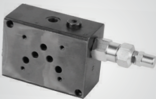
WINMAN singel-sicherheitsthalventil WINMAN NG10 valve manifolds
