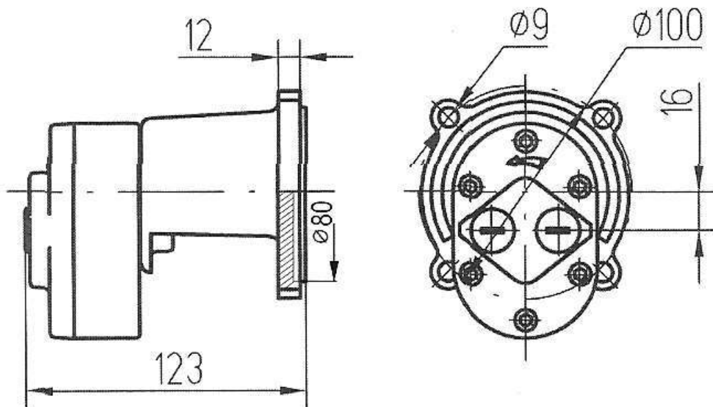
Габаритные и присоединительные размеры насосов ДБГ11-11, ДБГ11-11А
